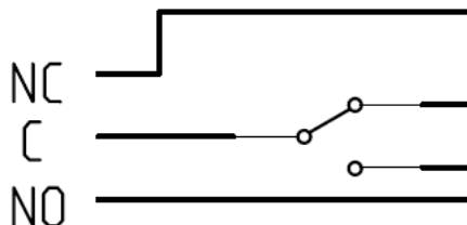
Рис. 3 - Схема подключения контактов одного реле
