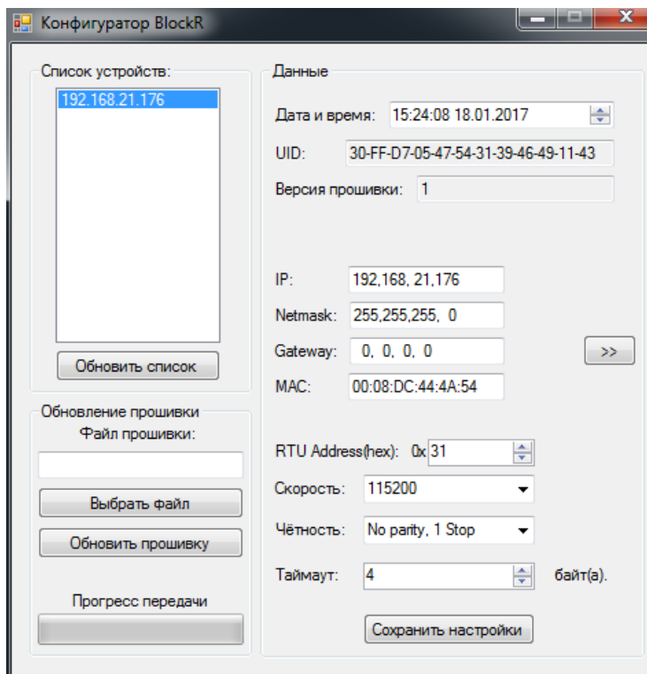
Рис.4 Основное окно сервисной утилиты PnktBlockR.exe.
