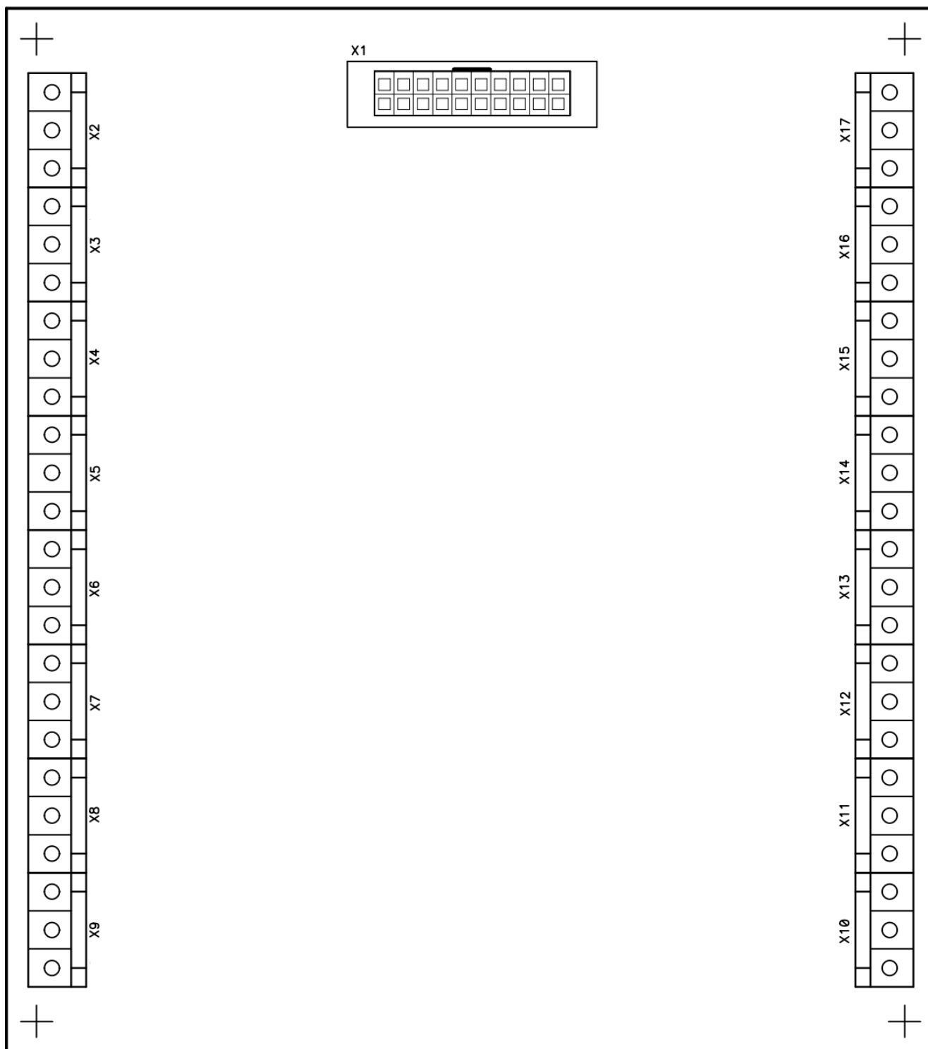
Рис.2 Коммутационные разъёмы модуля РМ-МР.
